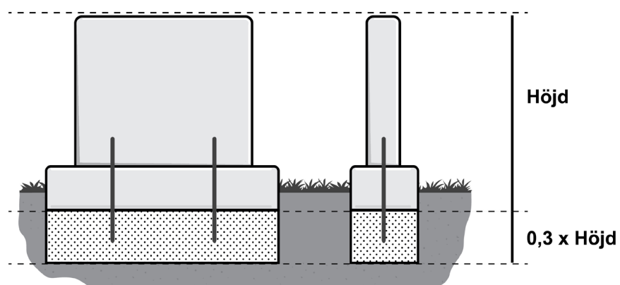
Figur 6. Synlig stensockel höjd 100 mm, dubbad i fundament av betong med genomgående dubbar.
