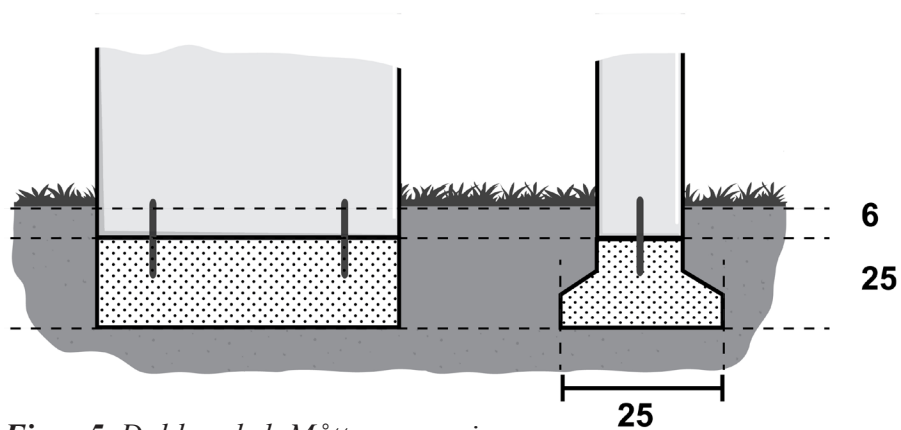
Figur 5. Dold sockel. Måtten anges i cm.
