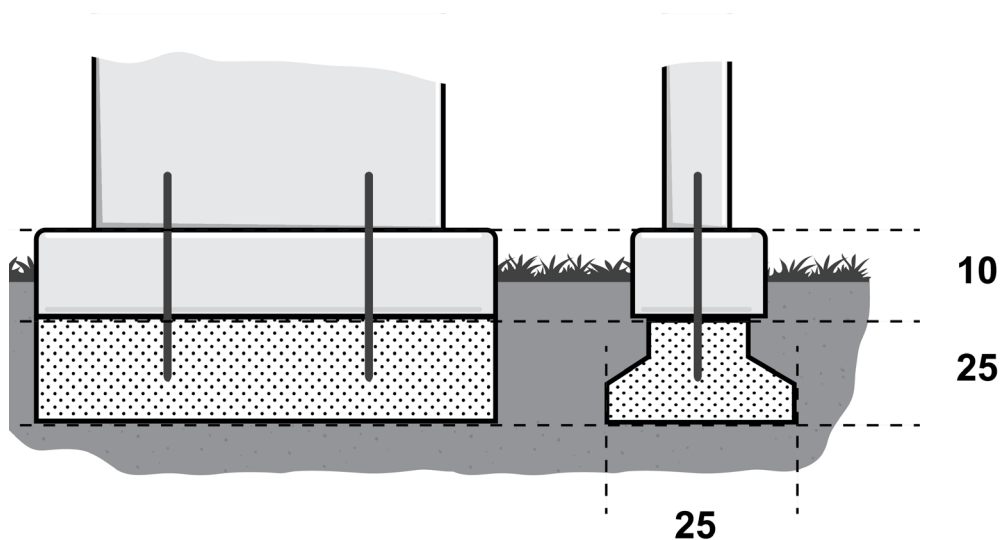
Figur 8. Synlig sockel, 100 mm hög, i granit. Måtten anges i cm.
