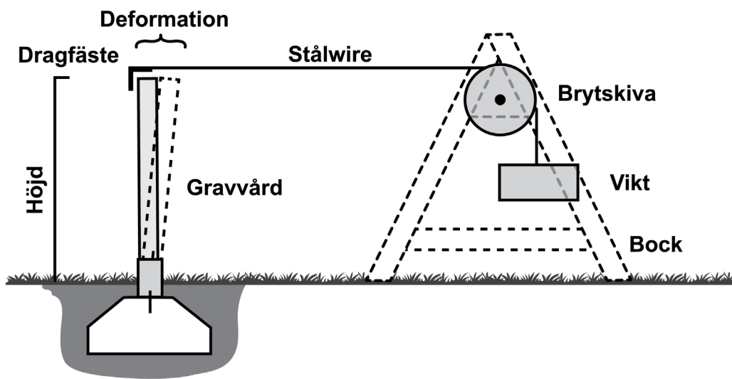
Figur 3. Skiss på konstruktion för statisk provning, elevation 1:20.
