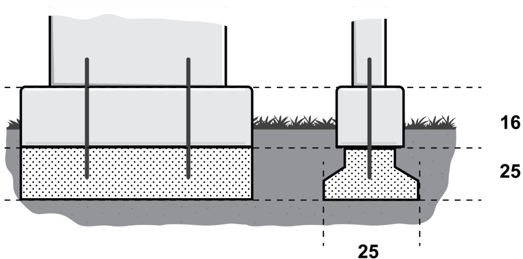
Figur 9. Synlig sockel, 160 mm, i granit. Måtten anges i cm.
