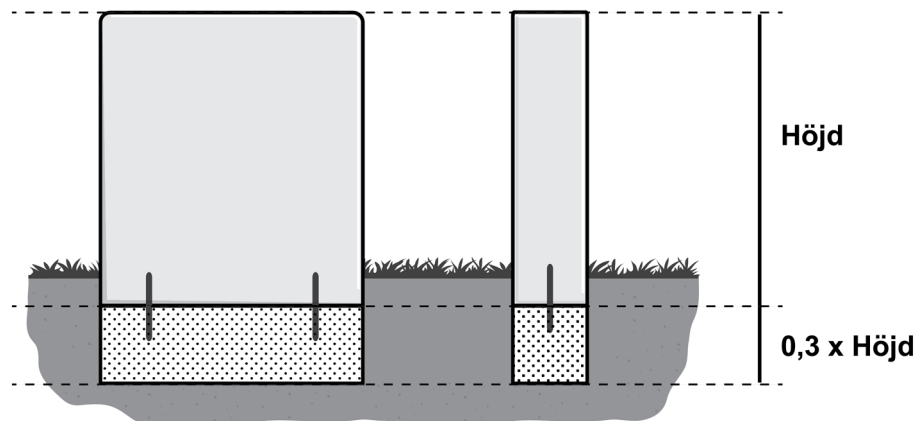
Figur 4. Dold sockel. Platsgjutet betongfundament under mark. Livstenen dubbas direkt i betongen. Om denna metod används kan monteringen ske i två steg. Först gjuts betongfundament med dubbar. När betongen härdat monteras livstenen.
